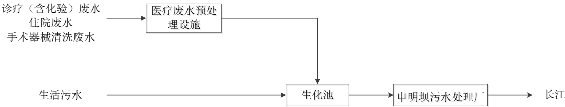
图 4-1 废水处理流程图
