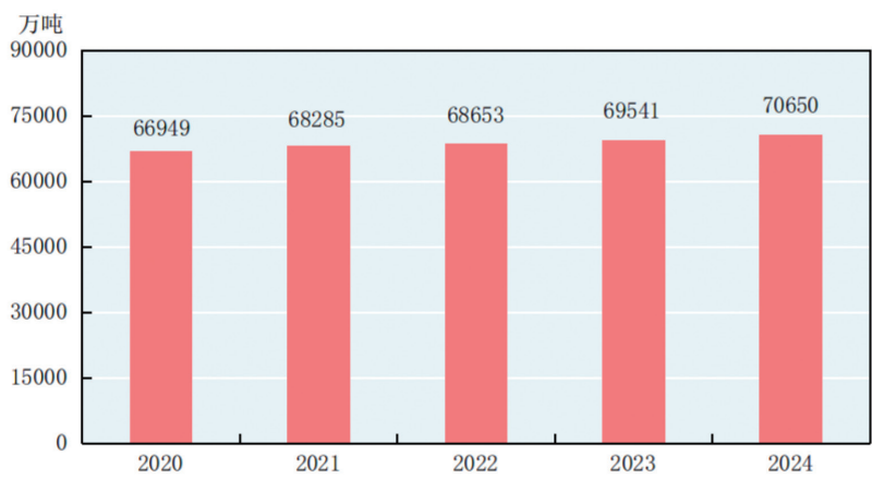
图 8 2020–2024 年粮食产量
