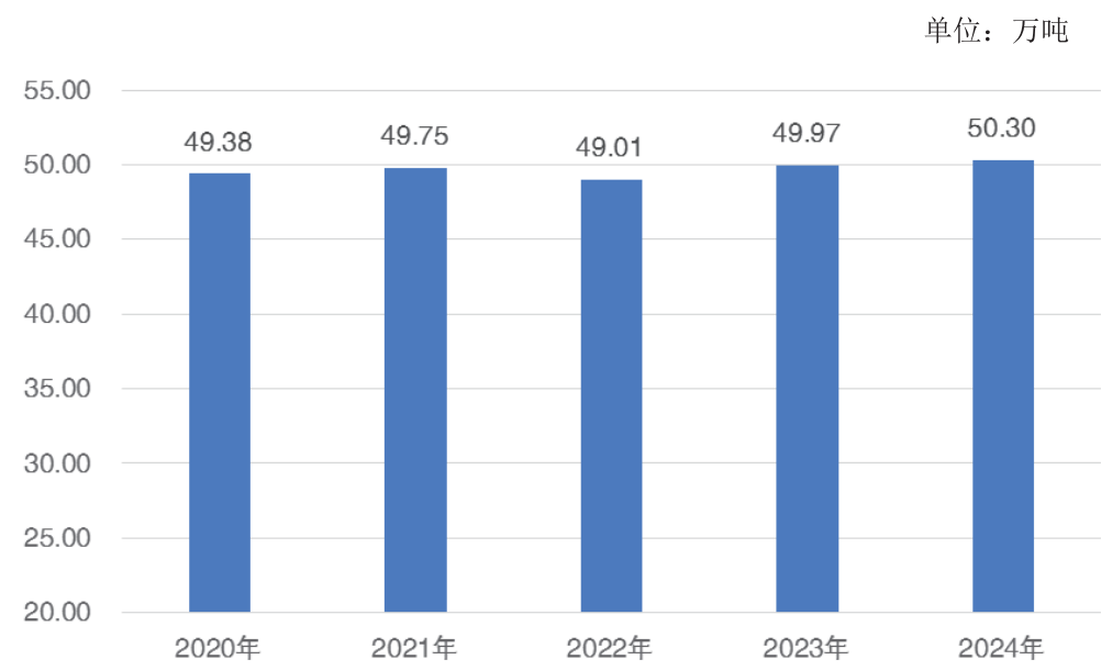
图 2 2020–2024 年粮食产量
