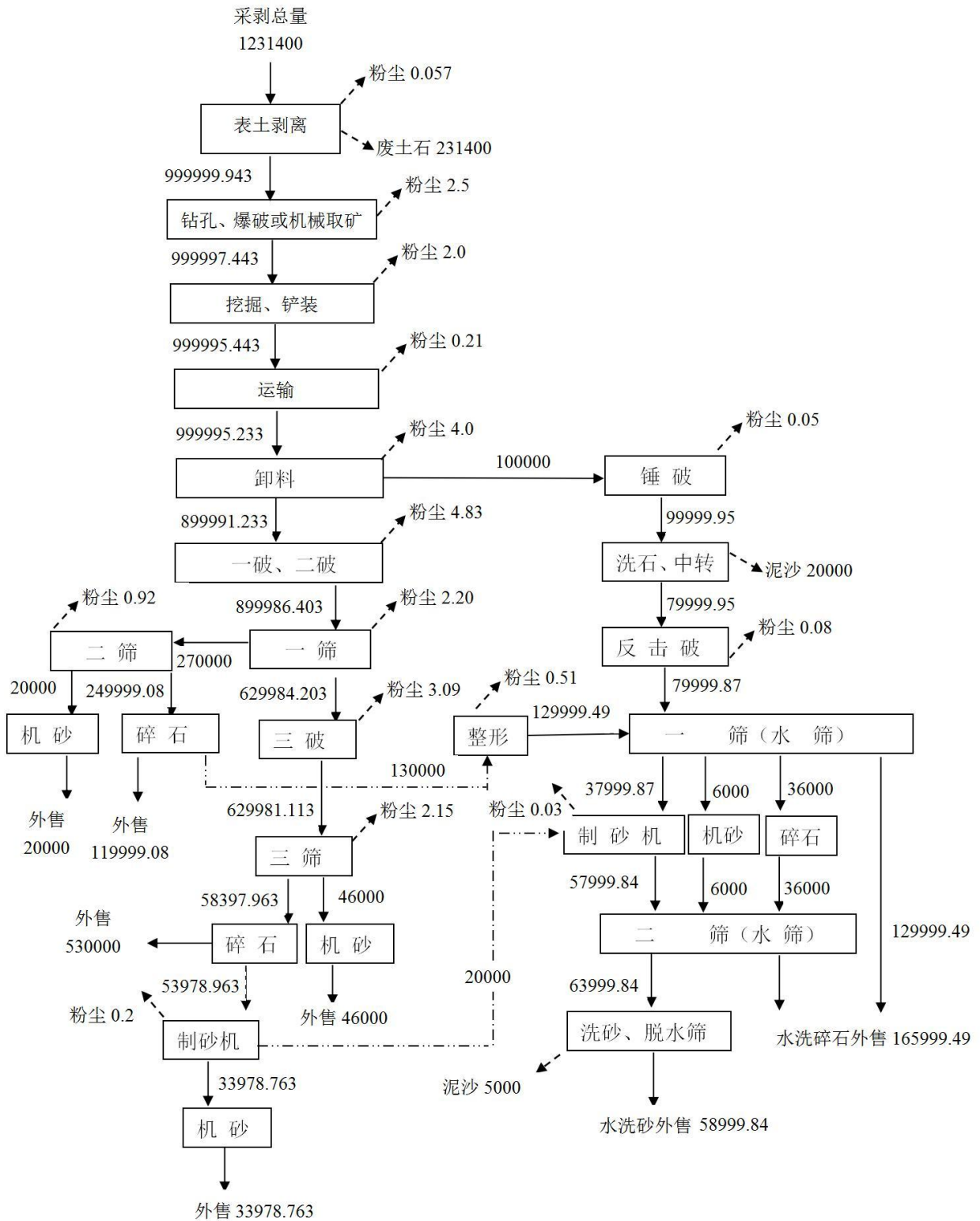
图 3.3-4 物料平衡图 单位: t/a
