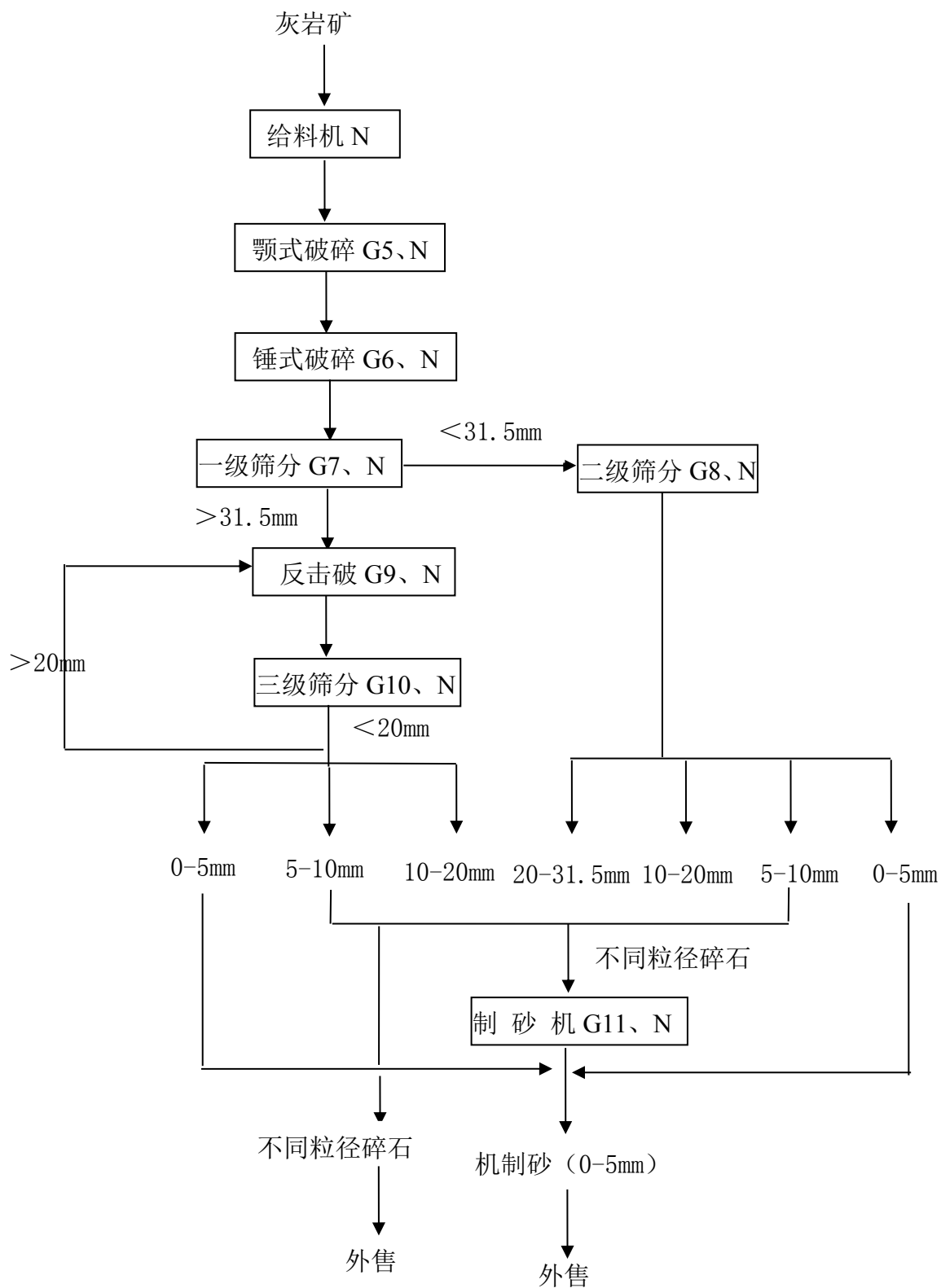
图 3.2-3 1#生产线（碎石生产线）工艺及产污环节流程图
